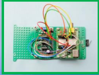
② Ichigojam を接続
